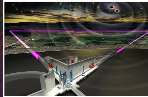
Einstein Telescope
