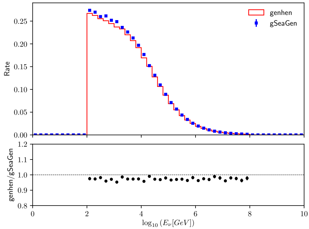
\nu_\mu NC
