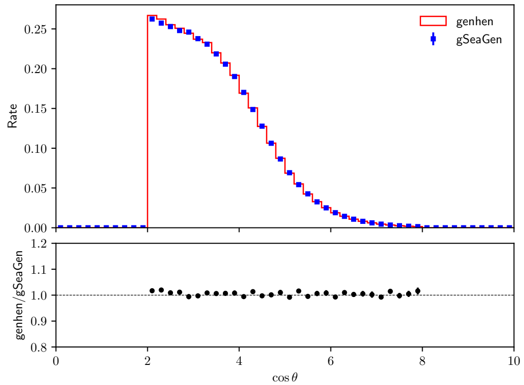
\nu_\mu NC
